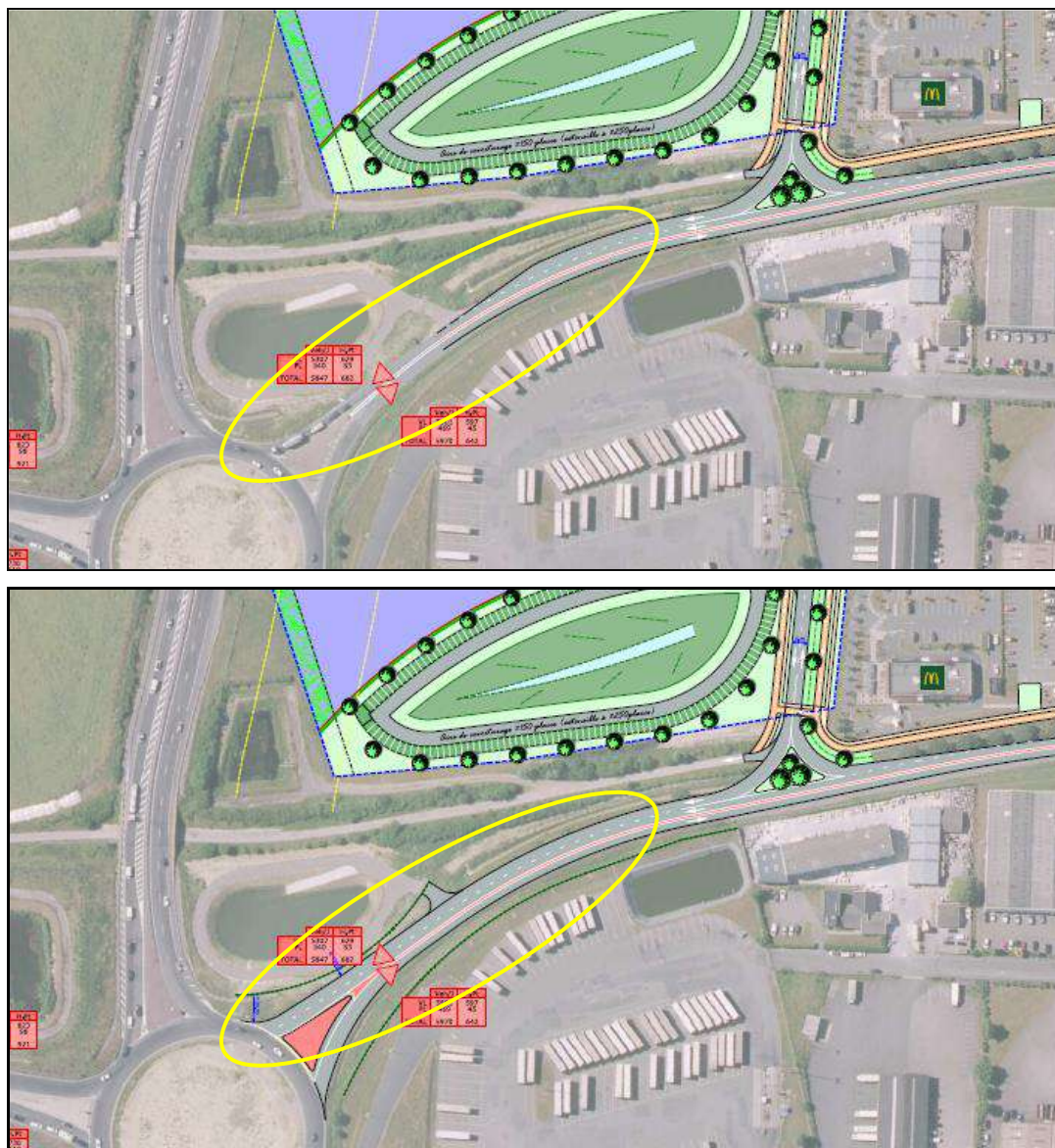
Document n° 87 : Variante au scénario 8 (doublement de la voirie de la Rue de la Rocade).
